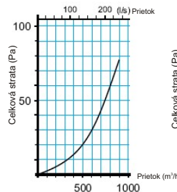
Tlaková strata (hadica koľajnice/m)
