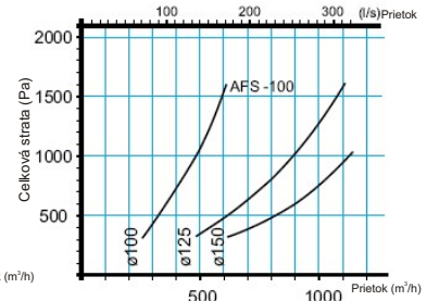
Tlaková strata (úplne rozbalená hadica, 5m)
