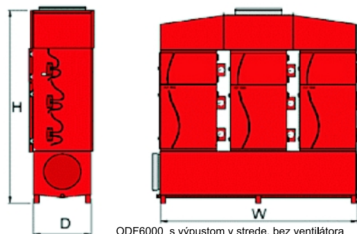
ODF6000 s výpustom v strede, bez ventilátora
